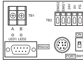
IAI SIO converter RCB-TU-SIO-A/B
